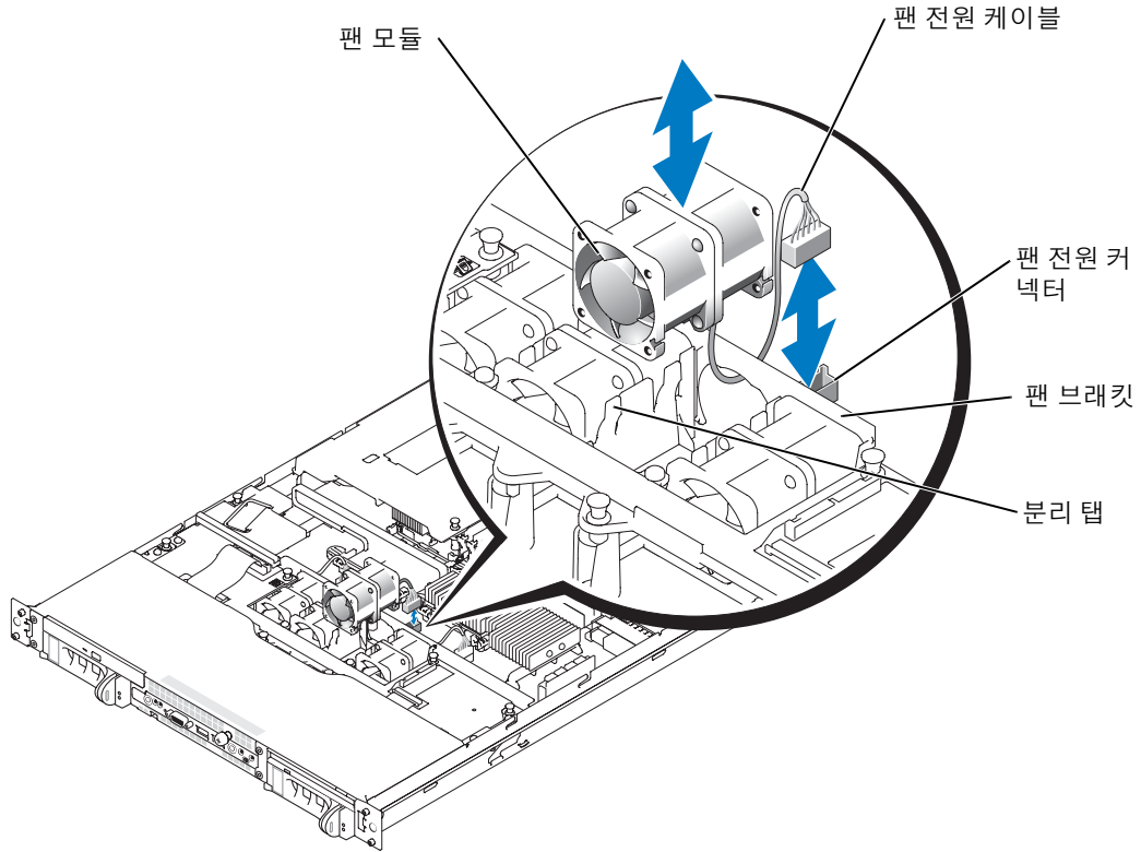
그림 1. 팬 모듈 분리 및 설치
