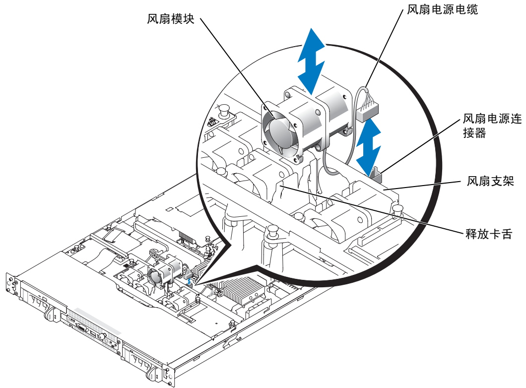
图 1. 卸下和安装风扇模块
