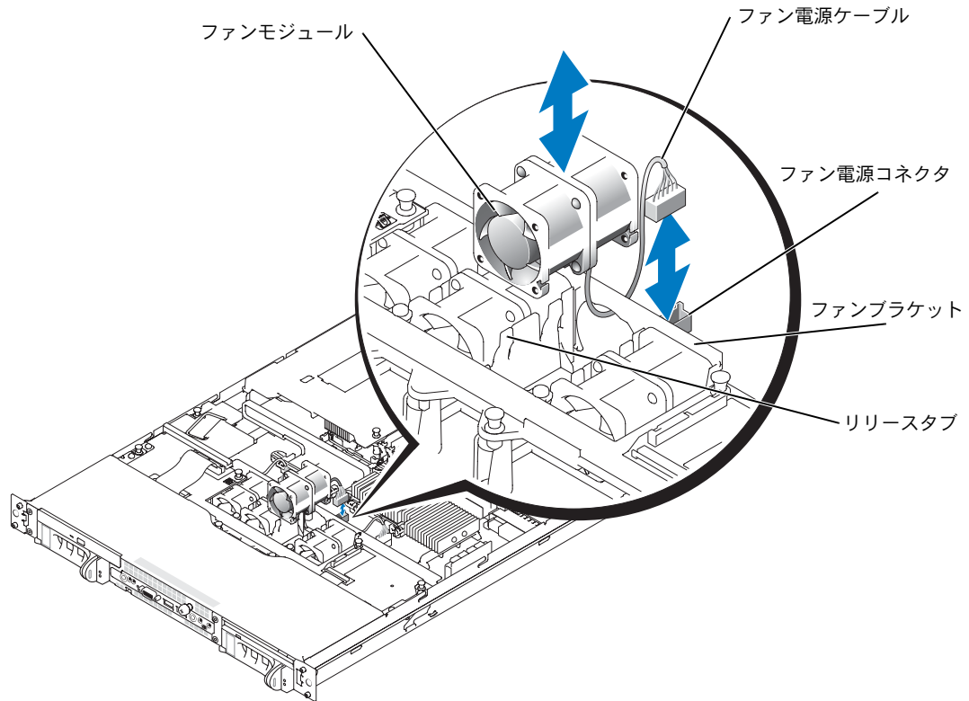
図 1. ファンモジュールの取り外しと取り付け
