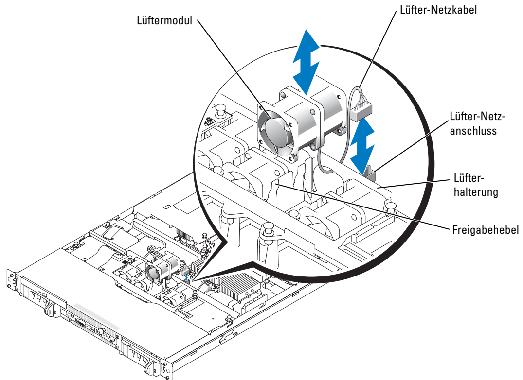
Abbildung 1. Lüftermodul ausbauen und einbauen
