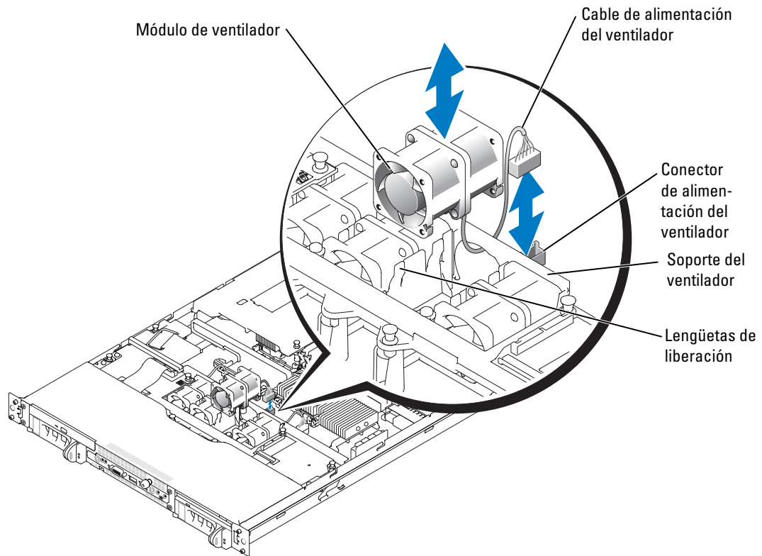
Figura 1. Extracción e instalación de un módulo de ventilador
