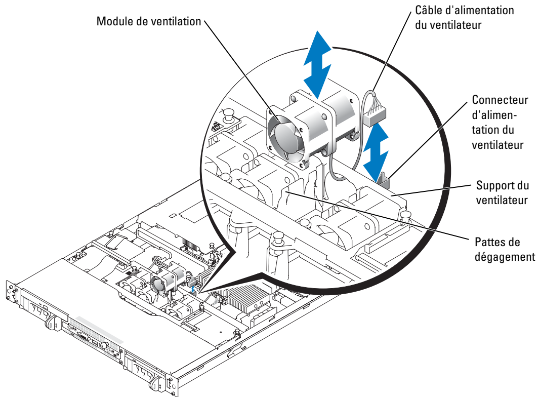
Figure 1. Retrait et installation d'un module de ventilation
